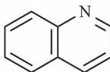
Quinoléine
