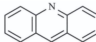
Quinoléine condensée
